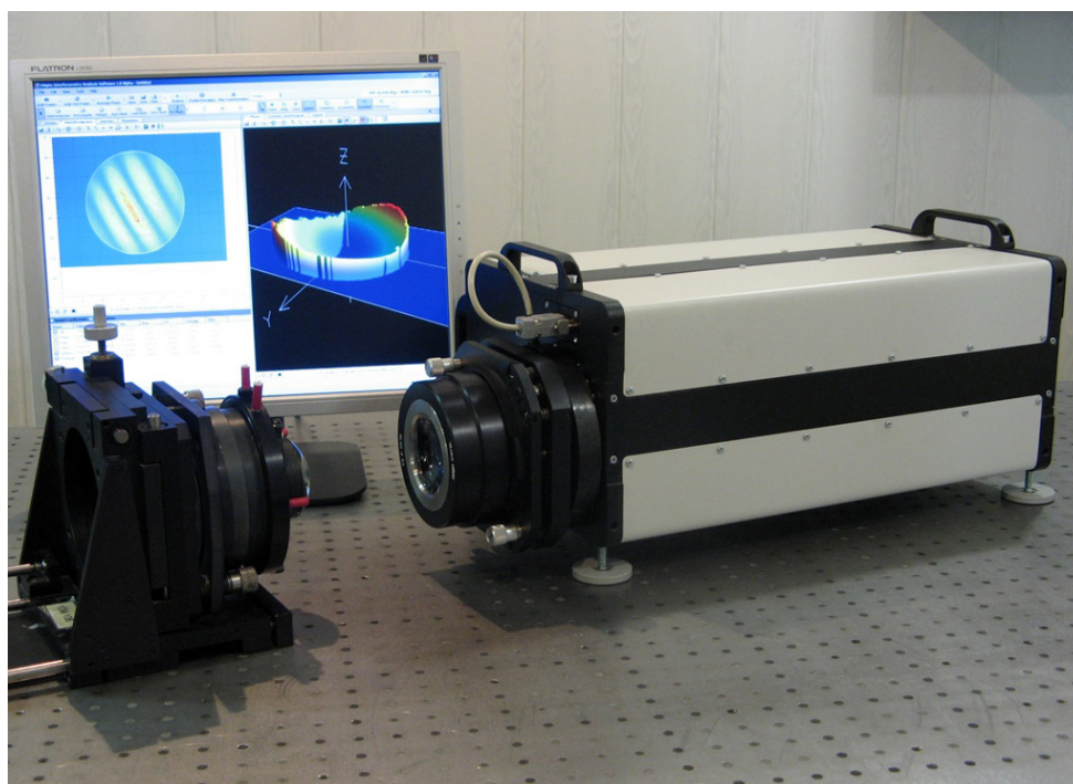
Лазерный интерферометр ФТИ-100PS
