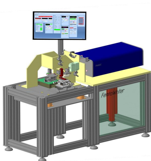
Рис. 2 Макет высокопроизводительной установки по выпуску в промышленных масштабах волоконно-оптических сенсоров
