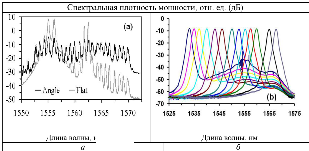
Рис. 1.3. a – спектр генерации волоконного лазера с линейкой ВБР-отражателей и рэлеевской СПОС (темная кривая) в сравнении с обычным ВКР-лазером с отражателем на торце волокна (серая кривая); б – перестройка спектра генерации СПОС-лазера с помощью АО фильтра
