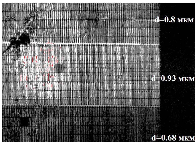
Рис. 2. Объект – поверхность синтезированной защитной голограммы, выполненной на основе дифракционных оптических микроструктур. Носитель – полимерная пленка толщиной 25 мкм. Периоды линий структуры 0.93 мкм, 0.8 мкм, 0.68 мкм, глубина структуры около 200 нм.
