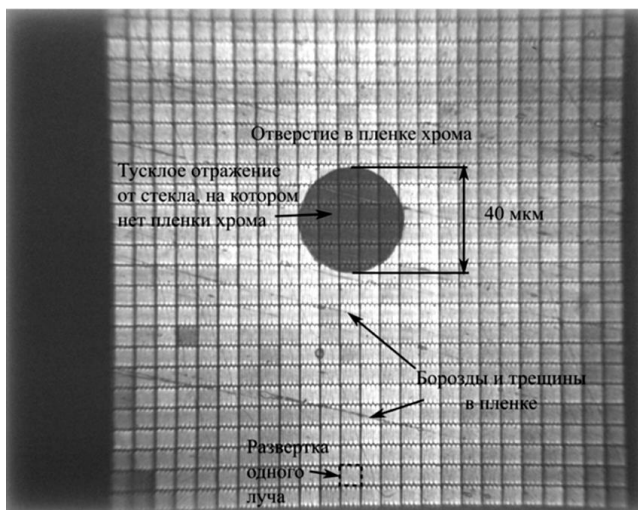
Рис. 1. Объект – круглое отверстие диаметром 40 мкм в пленке хрома на стеклянной подложке. Для наглядности показаны границы зон сканирования отдельных лучей.
