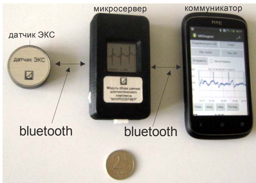
Макет системы мониторинга состояния сердечной деятельности пациента
