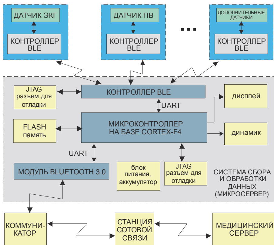
Схема работы диагностического комплекса для непрерывного мониторинга сердечной деятельности пациента
