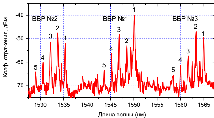
Рис. 12 — Спектры отражения массива ВБР, записанного в ММ ВС с градиентным профилем показателя преломления: ВБР №1 записана в центральной части сердцевины, а ВБР №2–3 с отступом \approx 10 мкм.
