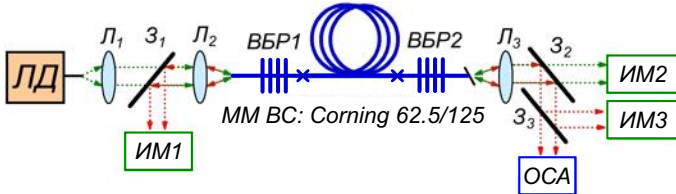
Рис. 13 — Схема ВКР-лазера на основе градиентного ММ ВС.
