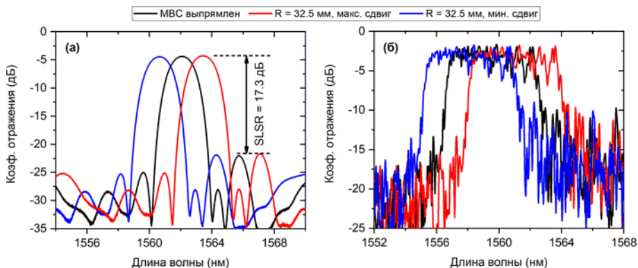
Рис. 9 — Спектры отражения линейно аподизированной (а) и чирпированной (б) ВБР, записанных в боковых сердцевинах 7-сердцевинного волоконного световода НЦВО РАН. Спектры измерялись для выпрямленного участка МВС (черный) и изогнутого (красный и синий).
