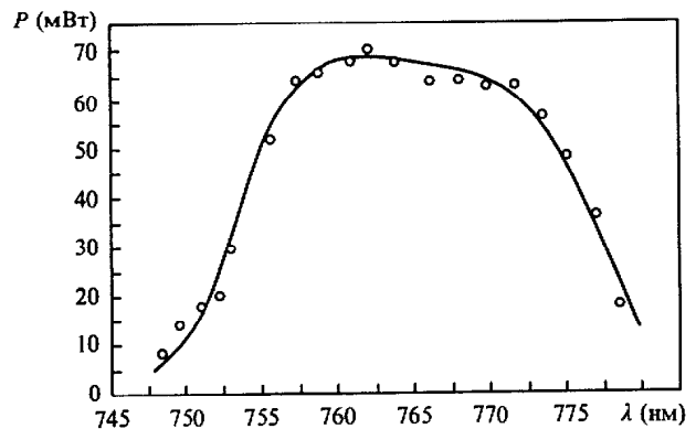
Рис.3. Зависимость средней мощности генерации P от длины волны излучения \lambda .
