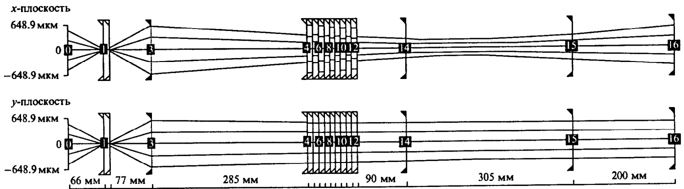
Рис.2. Ход лучей в резонаторе (пояснения даны в тексте).
