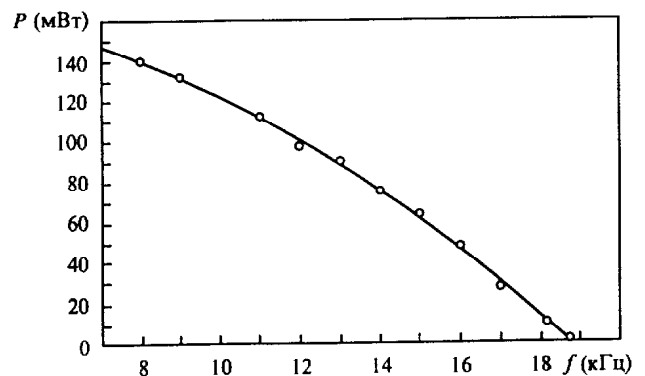
Рис.4. Зависимость средней мощности генерации P от частоты следования импульсов f .
